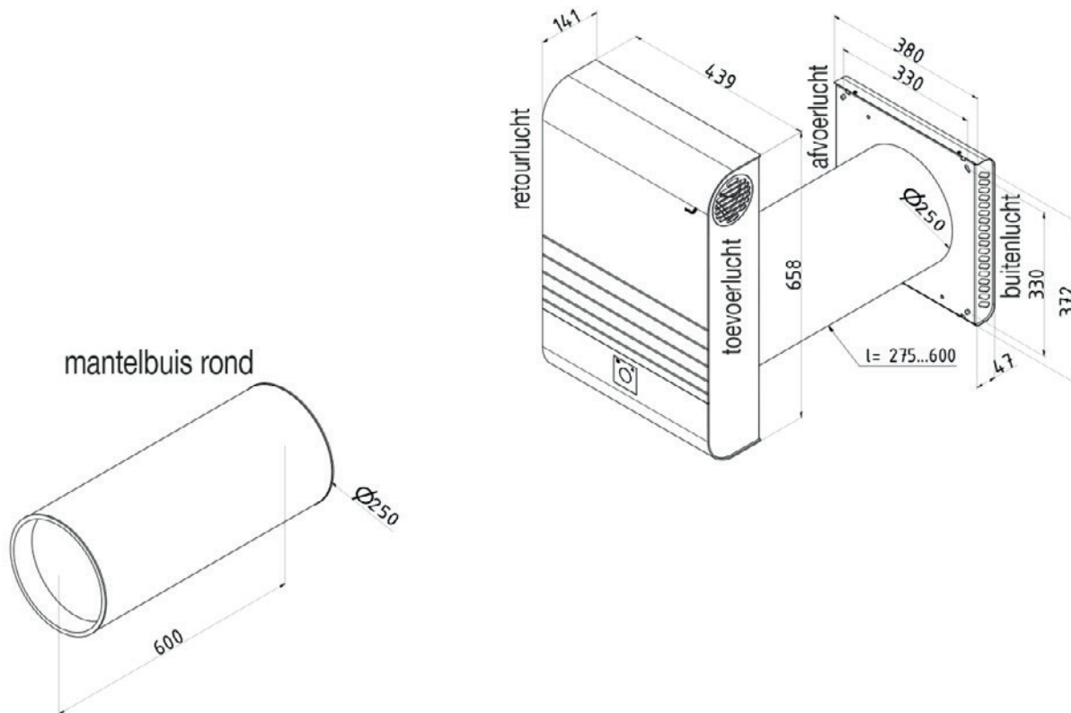
Afbeelding 2.0: ComfoAir 70 Maatschets
