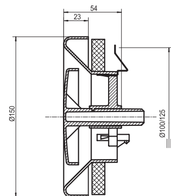
Afbeelding 1.0: Maatschets STK
