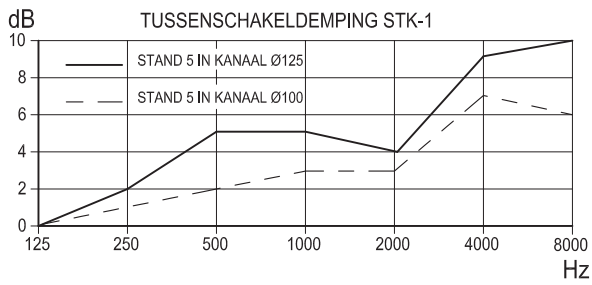
Afbeelding 2.0: Capaciteitsgrafieken
