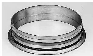
Type BF, met twee borgranden voor spiraalgefleste en gladde buizen
